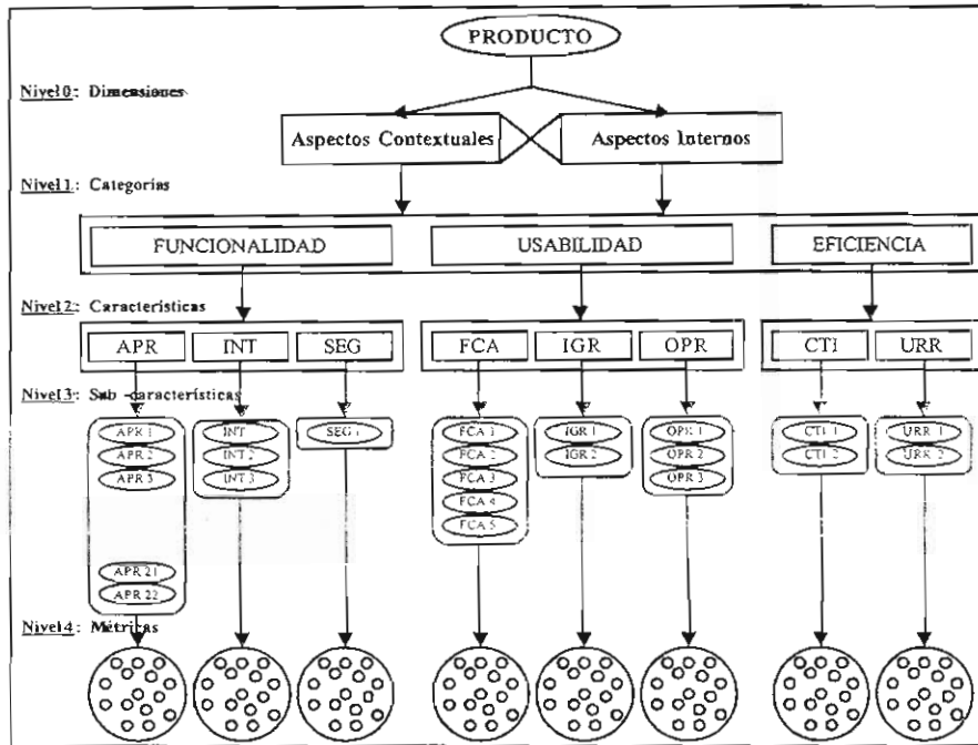
Fig. 1. Árbol Jerárquico de MOSCA+ [7].
